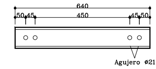
ALZADO
